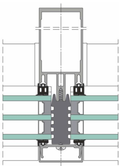
PRZEKRÓJ PRZEZ SŁUP FA 50N HI
