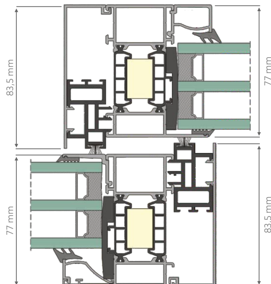
PRZEKRÓJ PRZEZ PRZYMYK DRZWI AUTOMATYCZNYCH TM 77HI
